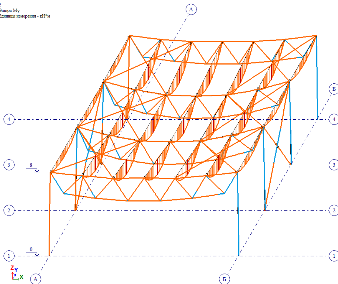
Минимальное усилие -2.11339; Максимальное усилие 37.8244
